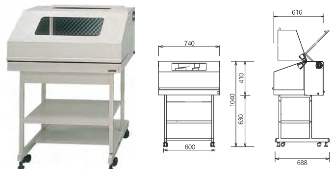
○本体寸法 (mm) : W740×D688×H1040
