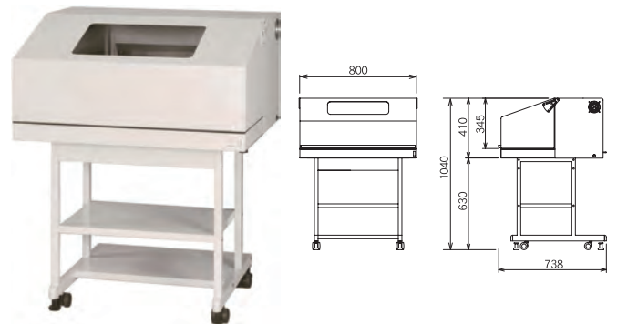
○本体寸法 (mm) : W800×D738×H1040
