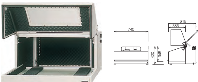
○本体寸法 (mm) : W740×D616×H420
